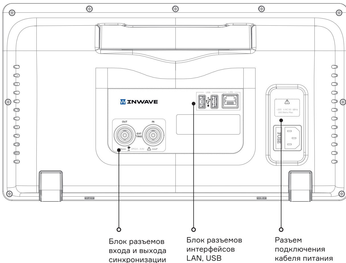
Рис. 2. Задняя панель
