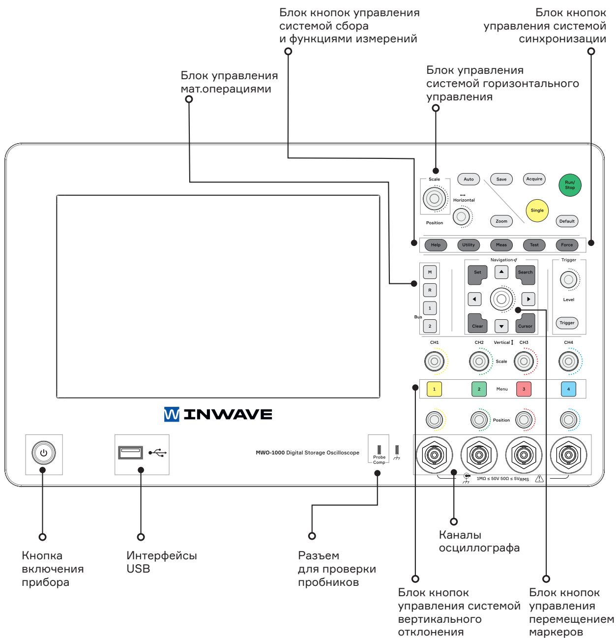
Рис. 1. Лицевая панель
